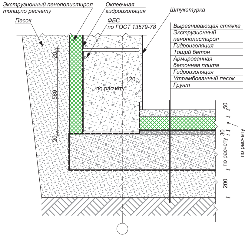
Фундаментная подушка
