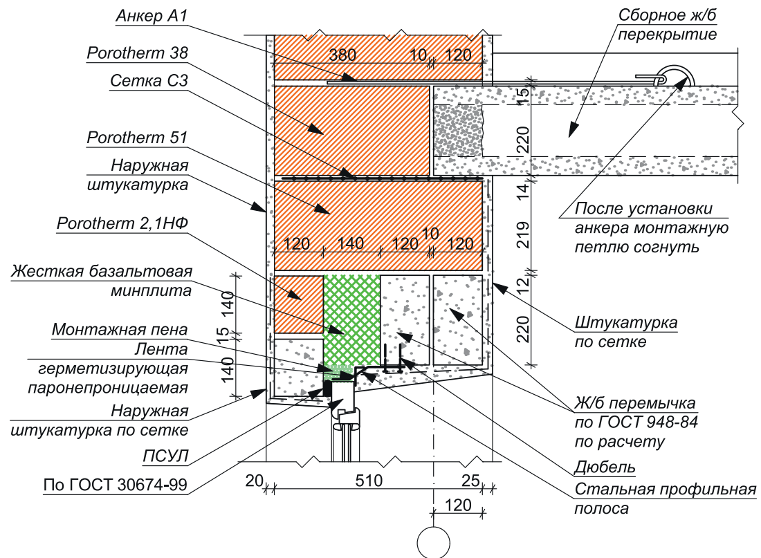
СТЕНА, ТИП 1. УВЕЛИЧЕННАЯ ВЫСОТА ЭТАЖА. УЗЛЫ (POROTHERM 44; 51)
