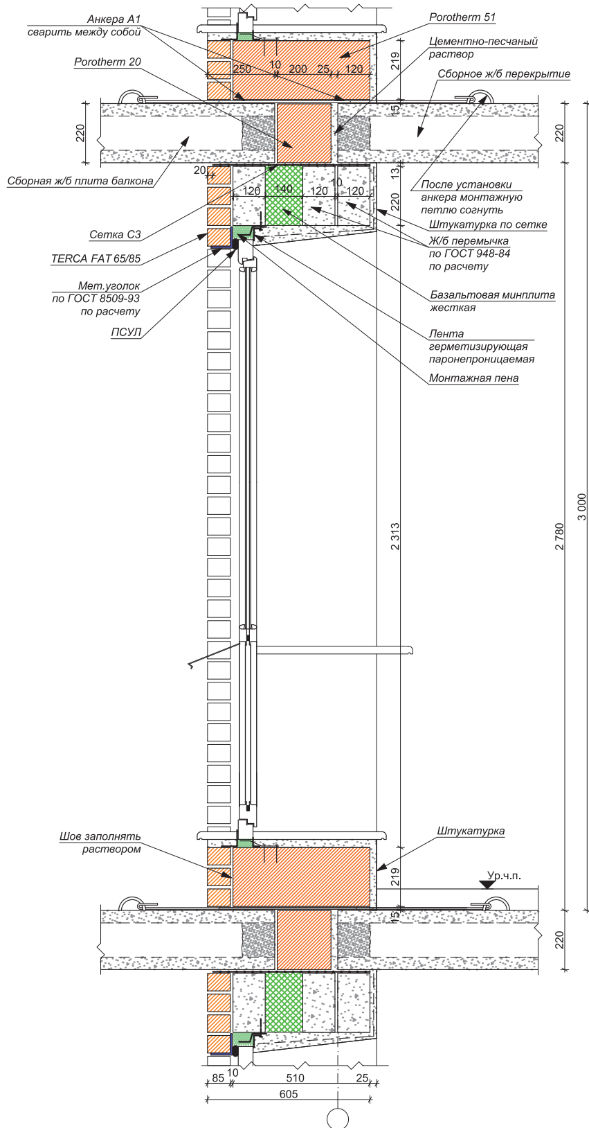
СТЕНА, ТИП 2. СЕЧЕНИЕ ПО БАЛКОННОЙ ДВЕРИ (ВАРИАНТ 2) (СБОРНОЕ ПЕРЕКРЫТИЕ. POROTHERM 51)
