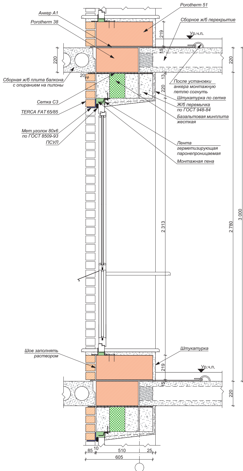
СТЕНА, ТИП 2. СЕЧЕНИЕ ПО БАЛКОННОЙ ДВЕРИ (СБОРНОЕ ПЕРЕКРЫТИЕ. POROTHERM 51)
